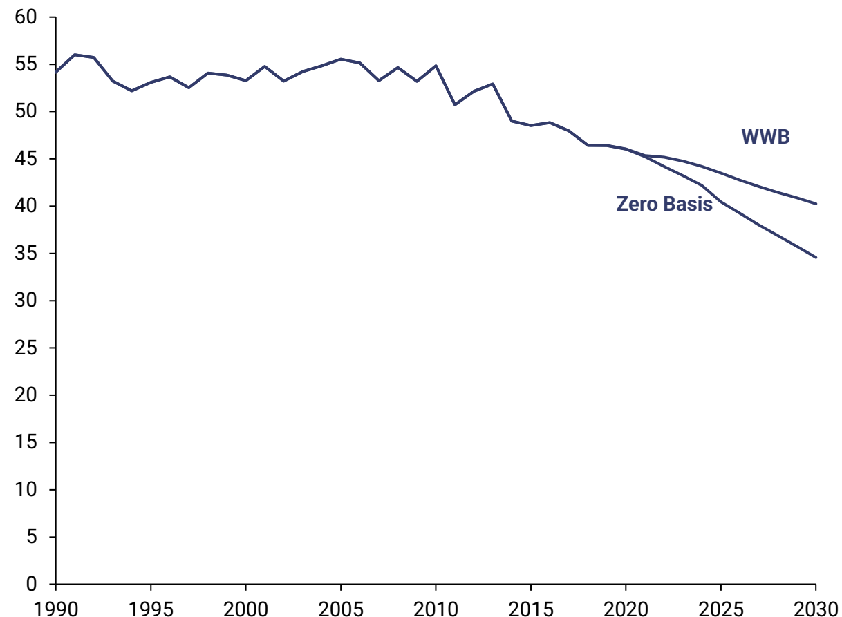
Das Zero Basis Szenario beschreibt eine schnellere Reduktion von Emissionen zum Erreichen der Klimaziele in 2050 1 (in MtCO 2 eq)
