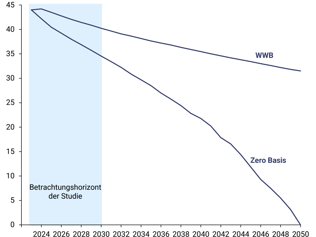
Auch nach 2030 steht die Schweiz vor grossen Herausforderungen 1,a (in Mt CO 2 eq)
