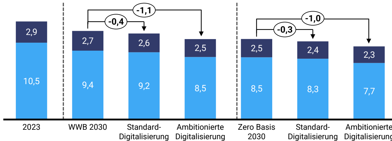
Im Verkehrssektor können bis zu 1,1 Mt CO 2 eq eingespart werden (in Mt CO 2 eq)
